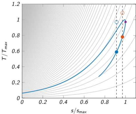
Rayleigh line ( Ts -diagram)
