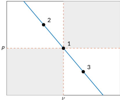
Rayleigh line ( p\nu -diagram)
