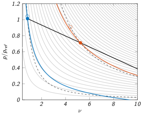
Rayleigh line ( p\nu -diagram)
