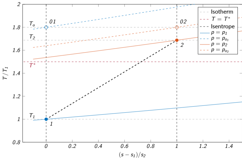
Normal shock ( Ts -diagram)
